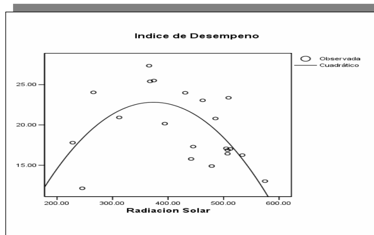
Figura 5: Gráficas de Estimación Curvilínea para el Índice de Desempeño, en función de la Radiación Solar diaria.
