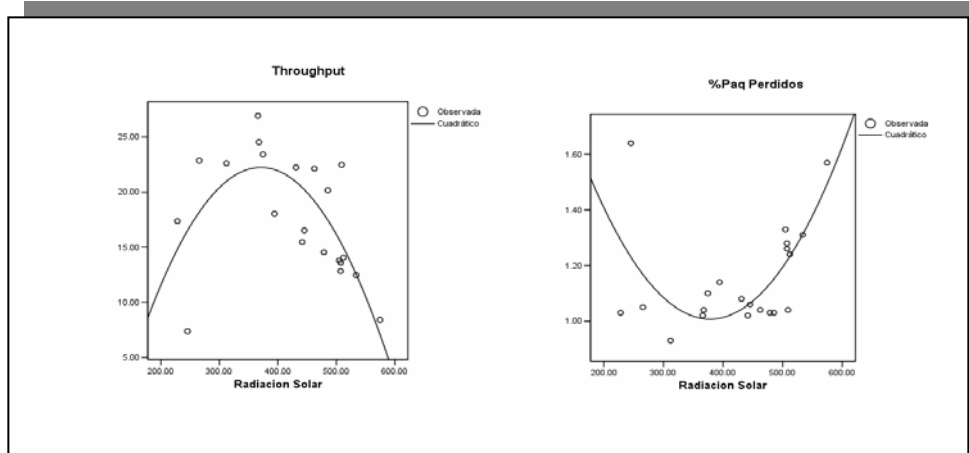
Figura 4: Gráficas de Estimación Curvilínea para el Throughput y el Porcentaje de Paquetes Perdidos, en función de la Radiación Solar diaria.
