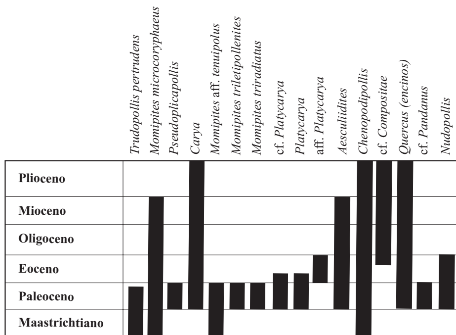
Figura 4. Asociación palinomórfica en los sedimentos continentales del nivel Po de la Figura 2 (Altamira-Areyán, 2002).
