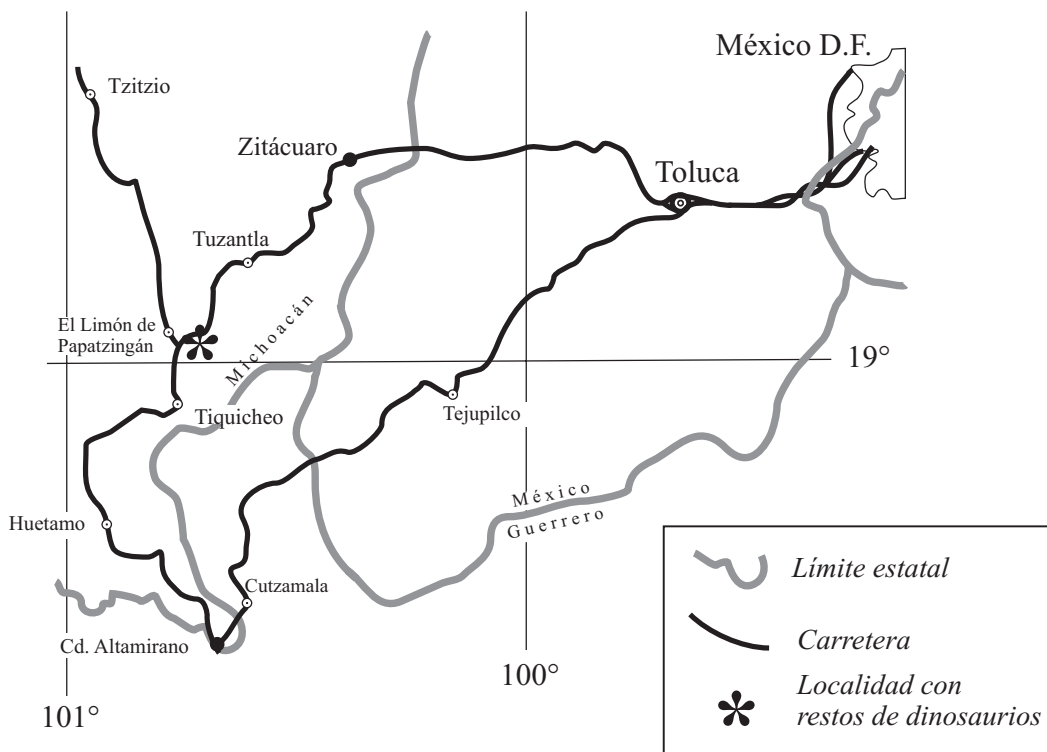
Figura 1. Mapa de localización del área de estudio (modificado de Altamira-Areyán, 2002).
