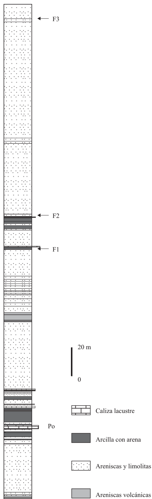
Figura 2. Una parte de la columna estratigráfica en la localidad Barranca Los Bonetes. Po: nivel de polen; F: nivel de restos de dinosaurios.
