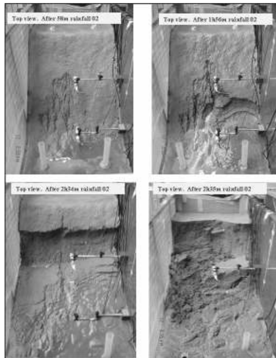
Figure 10. Photographs at various stages. Model No. 07 Figura 10. Fotografías en varias etapas. Modelo No. 07
