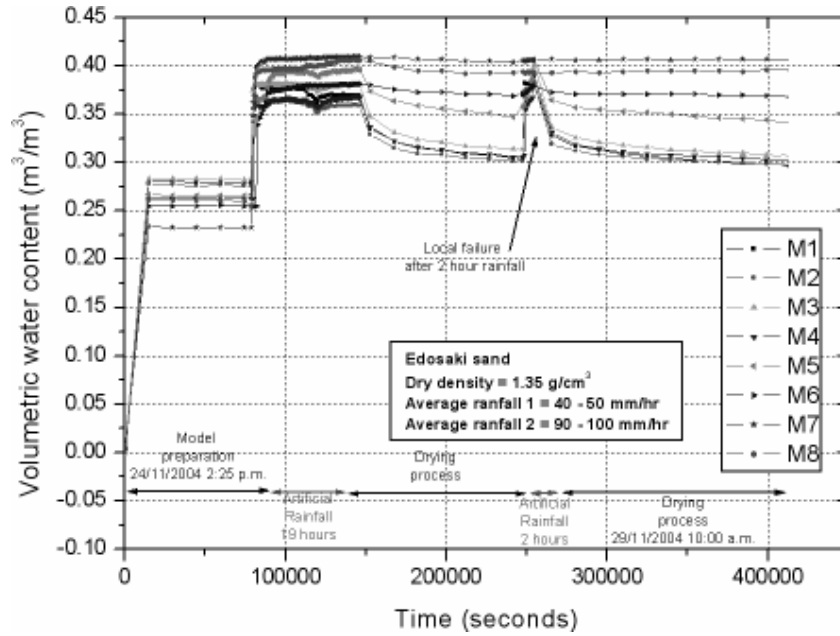
Figure 6. Time history of water content model No. 02 Figura 6. Registro histórico contenido de agua Modelo No. 02
